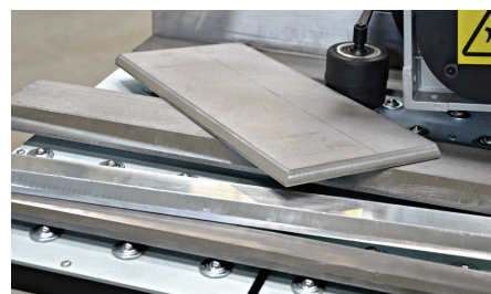
高品質な開先加工面
