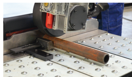
パイプ外径の開先加工も可能です
