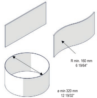
Klemme für Flacheisen (Option) DCS-0824-0037-00-0
