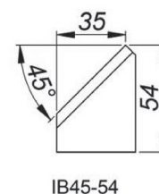
45° Nástrojový nůž pro vnitřní obrábění, Výška 54 mm [IB45/54] Číslo produktu: NOZ-000026
