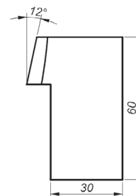
12° Speciální nůž Výška 60 mm Číslo produktu: NOZ-000086
