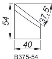
37.5° Obráběcí nůž, Výška 54 mm [B375/54] Číslo produktu: NOZ-000015
