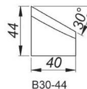
30° Obráběcí nůž, Výška 44 mm [B30/44] Číslo produktu: NOZ-000018
