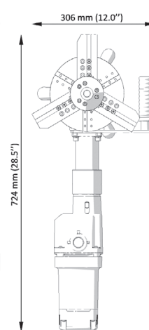
PRO-10 PB s elektrickým motorem
