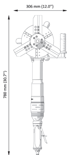
PRO-10 PB s pneumatickým pohonem
