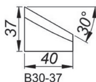
30° Obráběcí nůž, Výška 37 mm [B30/37] Číslo produktu: NOZ-000019
