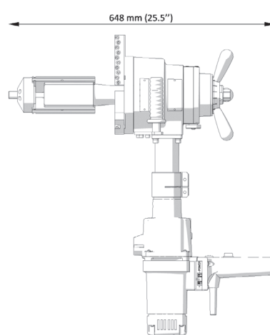
PRO-10 PB s elektrickým motorem
