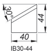
30° Nástrojový nůž pro vnitřní obrábění, Výška 44 mm [IB30/44] Číslo produktu: NOZ-000023
