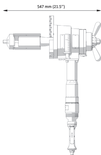
PRO-10 PB s pneumatickým pohonem
