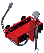
Rohrbefestigung DMP 251 für Rohre mit einem Durchmesser von 80-250 mm Produktcode: PDS-0110-03-00-01-0
