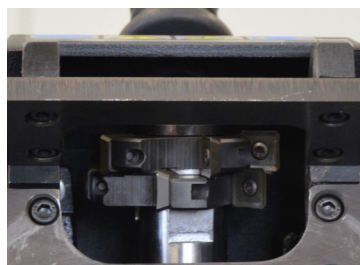
2 roterende fasehoder, som hver bruker fem firesidige vendeskjær
