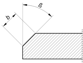
Tegning 1 Avfasingsdimensjoner; maksimal fasebredde avhengig av vinkelen
