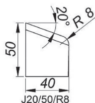
20° Schneidplatte für J-Fasen, Höhe 50 mm, Radius 8 mm [J20/50/R8] Produkt-Code: NOZ-000016
