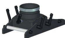
Aufsatz zum Entfernen von Schweißnähten an zylindrischen Längsflächen (min. ID 350 mm) mit einer Neigungswinkeleinstellung bis zu 15 Grad PRW-0761-12-00-00-0
