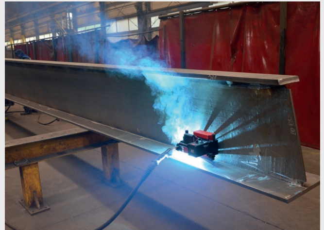
SCHWEISS-TRAKTOREN / BAUTEILFAHREND
