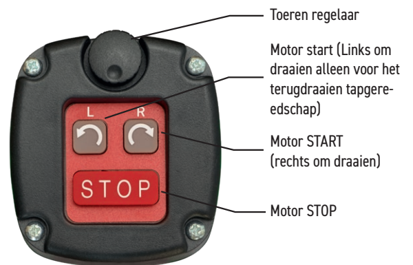
Intuïtief bedieningspaneel bovenop de boormachine
