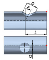
Gaură rotundă cu șanfren
