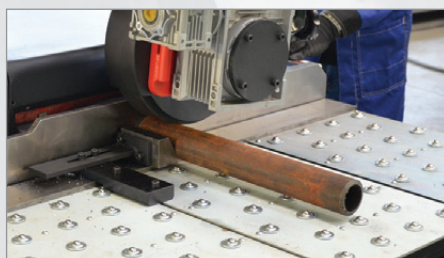
Possibility of pipe OD beveling
