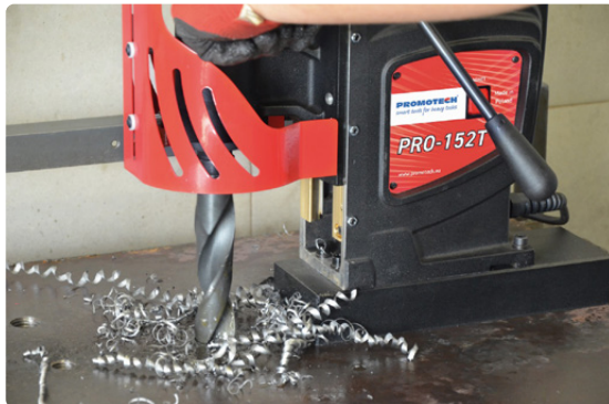
Foratura con punte elicoidali max 47 mm Corsa 260 mm
