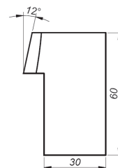
12° Outil de coupe special, Hauteur 60 mm Référence: NOZ-000086
