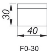
Outil de dressage des bords, Hauteur 30 mm [F0/30] Référence: NOZ-000017
