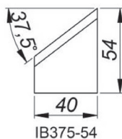
37.5° Outil de coupe chanfrein interne, Hauteur 54 mm [IB375/54] Référence: NOZ-000024
