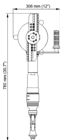
PRO-10 PB avec moteur pneumatique
