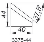
37.5° Outils de coupe chanfrein, Hauteur 44 mm [B375/44] Référence: NOZ-000020
