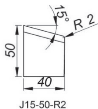
15° Outil de coupe chanfrein en "J", Hauteur 50 mm, Rayon 2mm [J15/50/R2] Référence: NOZ-000022
