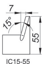
15° Outil de coupe rectification interne, Hauteur 55 mm [IC15/55] Référence: NOZ-000001
