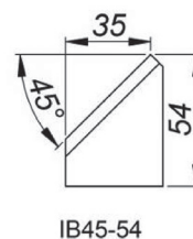
45° Outil de coupe chanfrein interne, Hauteur 54 mm [IB45/54] Référence: NOZ-000026
