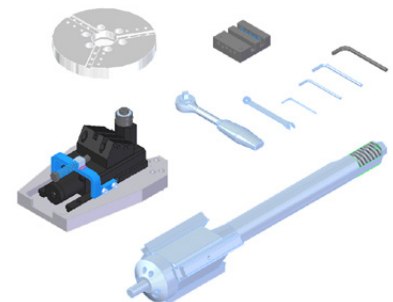
Kit pour tube ovalisé comprenant un grand mandrin pour un diamètre intérieur de tube de 126 à 296 mm et un disque pour trois porte-embouts. Référence: PRK-0807-07-00-00-0
