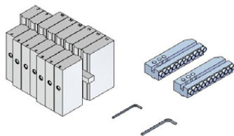
Kit d'extension pour diamètre extérieur jusqu'à 355 mm (14") comportant 2 porte-outils allongés et les mâchoires 7, 8, 9, 10, 11 Recommandé pour une épaisseur de paroi de tube jusqu'à 7 mm (0.26") Référence: ZST-0807-08-00-00-0
