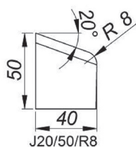
20° Outil de coupe chanfrein en "J", Hauteur 50 mm, Rayon 8mm [J20/50/R8] Référence: NOZ-000016
