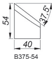
37.5° Outils de coupe chanfrein, Hauteur 54 mm [B375/54] Référence: NOZ-000015
