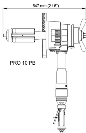
PRO-10 PB avec moteur pneumatique
