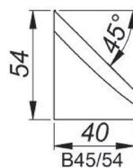
45° Outils de coupe chanfrein, Hauteur 54 mm [B45/54] Référence: NOZ-000021
