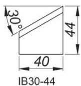
30° Outil de coupe chanfrein interne, Hauteur 44 mm [IB30/44] Référence: NOZ-000023
