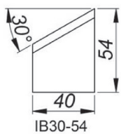
30° Outil de coupe chanfrein interne, Hauteur 54 mm [IB30/54] Référence: NOZ-000025
