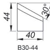
30° Outils de coupe chanfrein, Hauteur 44 mm [B30/44] Référence: NOZ-000018
