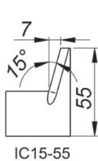
15° Internes Kalibrierwerkzeug, Höhe 55 mm [IC15/55] Produkt-Code: NOZ-000001
