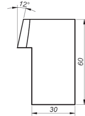
12° Spezielle Schneidplatte, Höhe 60 mm Produkt-Code: NOZ-000086
