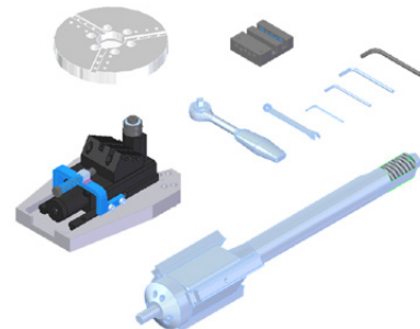
Ovales Aufnahmeset inkl. großem Dorn für Rohr-ID \varnothing 126 - 296 mm (5 bis 11-5/8") und Spindelteller für zwei Werkzeughalter Produkt-Code: PRK-0807-07-00-00-0
