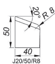
20° Schneidplatte für J-Fasen, Höhe 50 mm, Radius 8 mm [J20/50/R8] Produkt-Code: NOZ-000016
