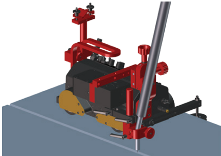
Soudage bout à bout avec oscillateur
