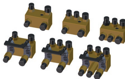
Porta torcia di precisione Ø 30 mm (1,18") UCW-0475-59-00-00-0
