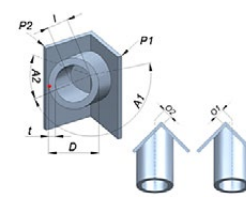
Rohr-Eckstoß
