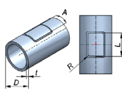
Rechteck-Ausschnitt
