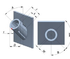
Rohr-Knotenblech
