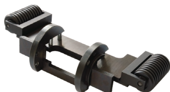
Attacco per spianatura (0°) (consente la smussatura con angolo zero) Codice prodotto: ZSP-0075-32-00-00-1
