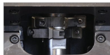
2 teste di fresatura rotanti, ciascuna contenente cinque inserti intercambiabili a 4 taglienti
