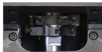
2 roterende freeskoppen met elk vijf 4-zijdige wisselplaten
