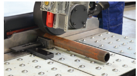
Possibility of pipe OD beveling
