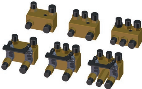
Präziser Brennerhalter mit Winkel- und Höhenverstellung UCW-0475-08-00-00-0
