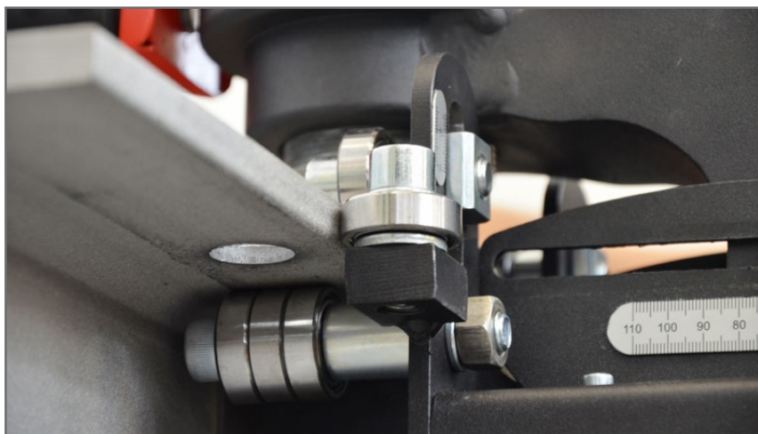
Permite um movimento linear suave e eficiente ao longo da peça de trabalho.
