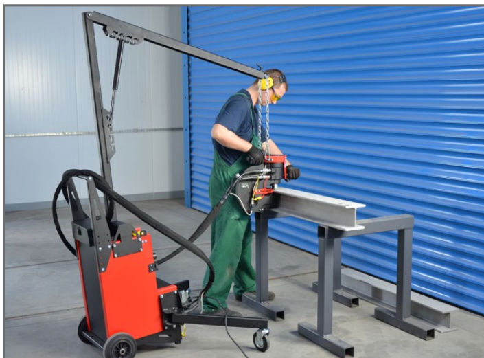
Braço de elevação e 2 apoios com rodas permitem uma fácil manipulação do punção e do gerador hidráulico como unidade única.
