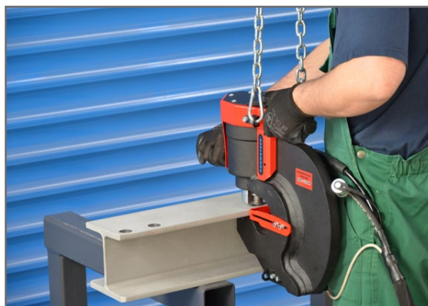
Braço de elevação e 2 apoios com rodas permitem uma fácil manipulação do punção e do gerador hidráulico como unidade única.
