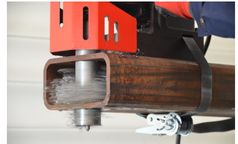
Startpunkt der Bohrung bis 50 mm unter dem Niveau des Bohrsockels mit 100 mm langem Fräser
