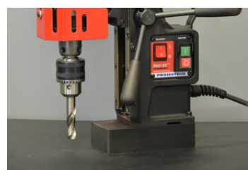
Adapter 3/4" x 1/2" 20 UNF, Bohrfutter 1/2" 20 UNF Spiralbohrer bis zu \Phi 16.0 mm (DIN 1897)
