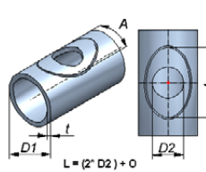
Coupe renforcement
