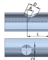
Trou rond avec chanfrein
