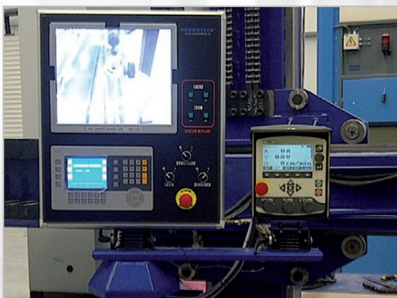
Manipolatore a bandiera standard con ESAB Aristo 1000 AC / DC
