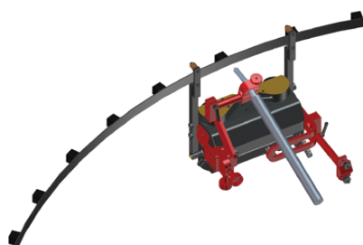
Nastavitelný vodící přípravek. Umožňuje i paralelní vedení s hranou. UST-0466-53-00-00-0
