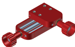
Křížovy posuv 0-76 mm (0-3") nahoru-dolů 0-35 mm (0-1.38") doleva-doprava ZSP-0466-46-00-00-1
